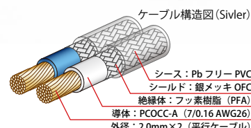
ケーブル構造図 (Silver)
